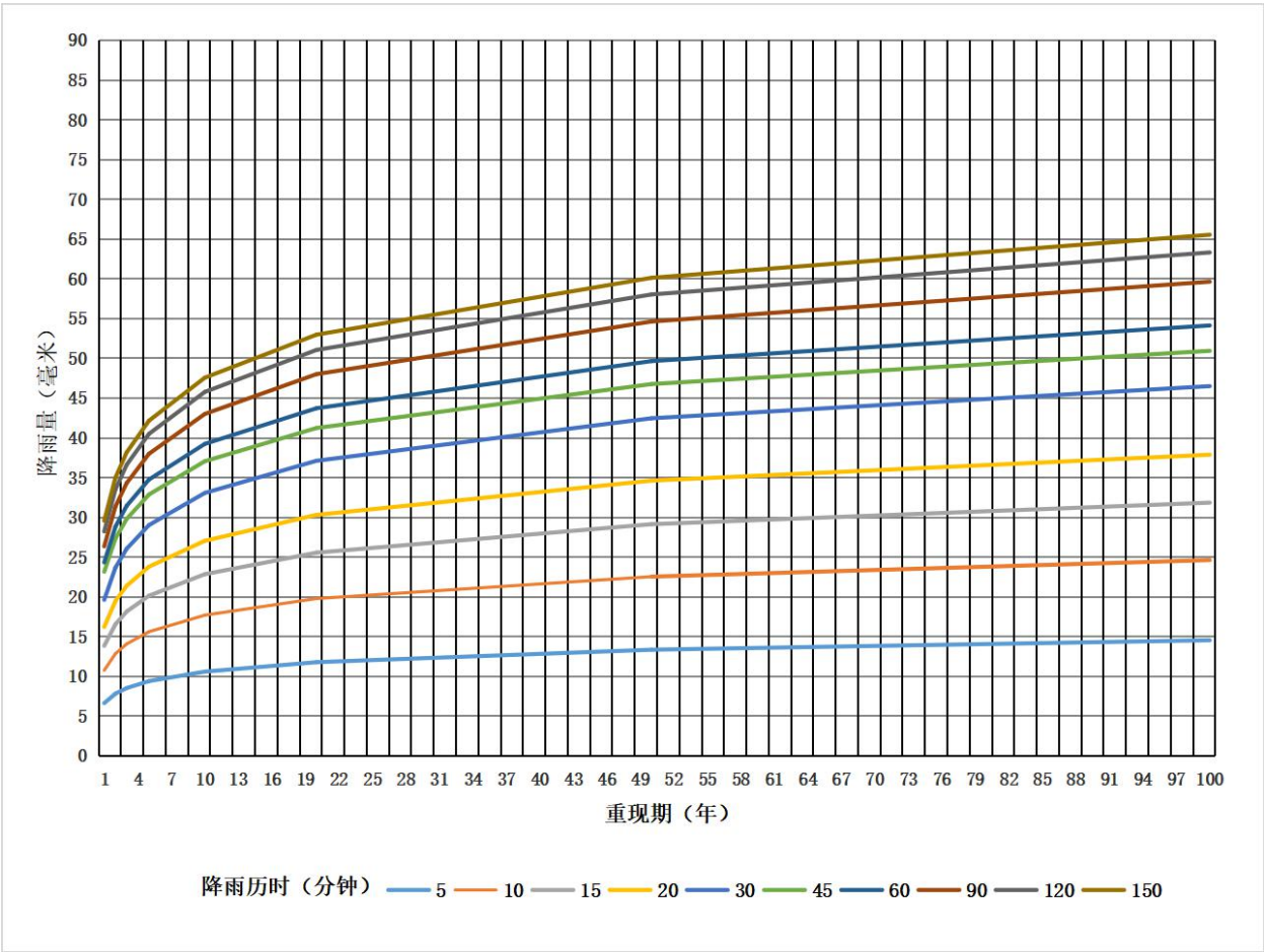
图 A. 2 临翔区不同历时降雨曲线
