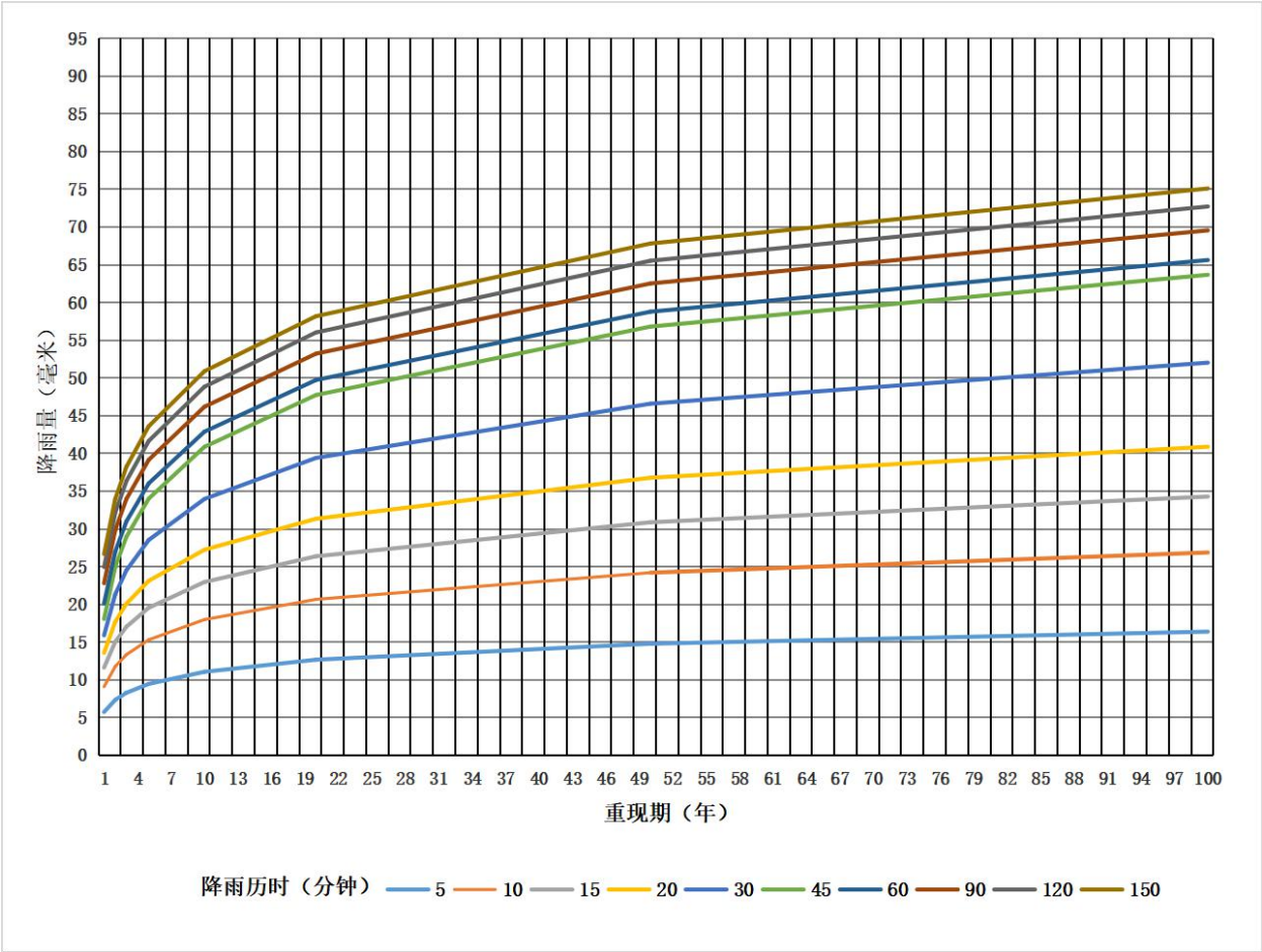
图 A. 16 双江县不同历时降雨曲线
