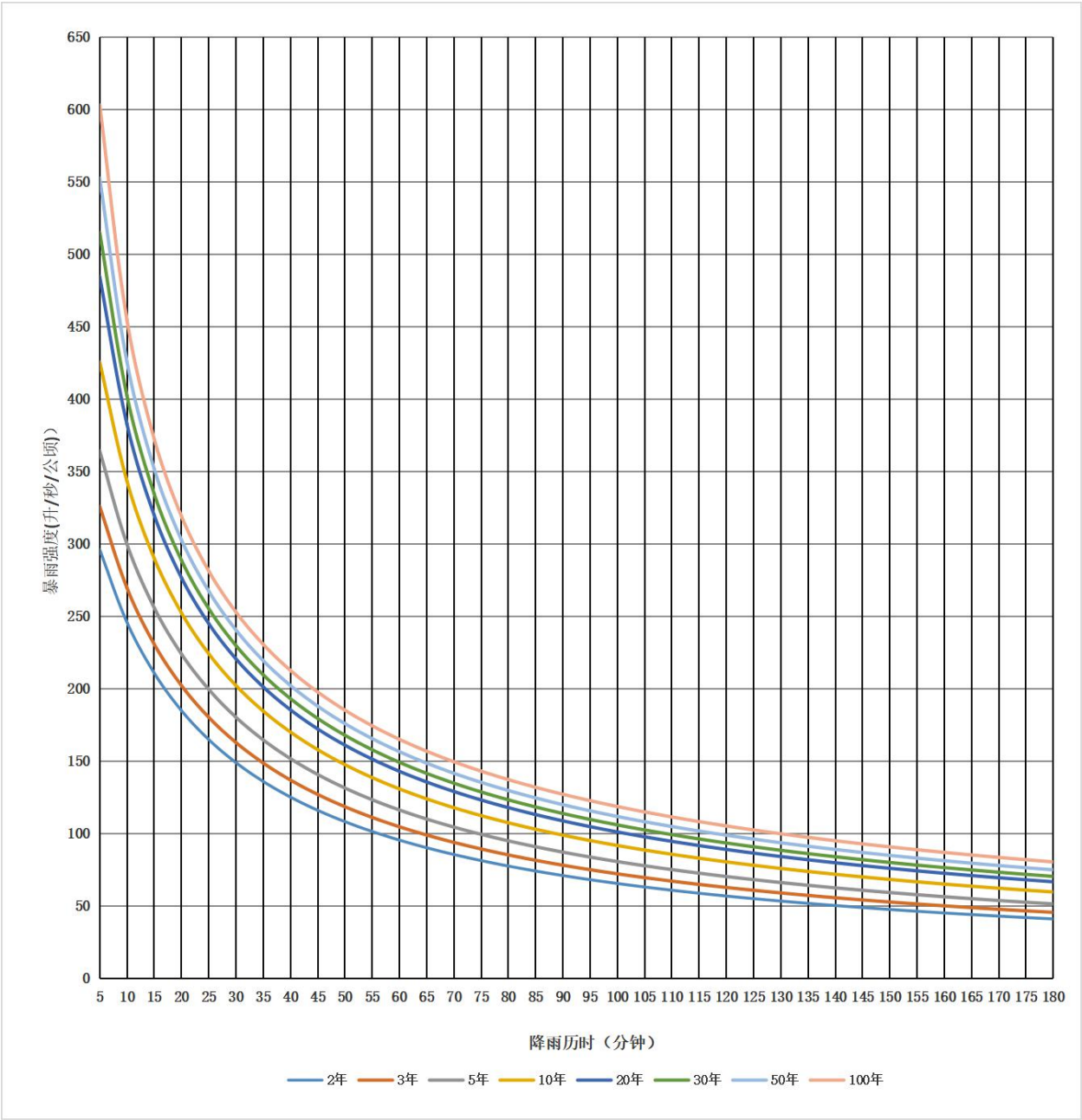
图 A. 11 耿马县暴雨强度曲线
