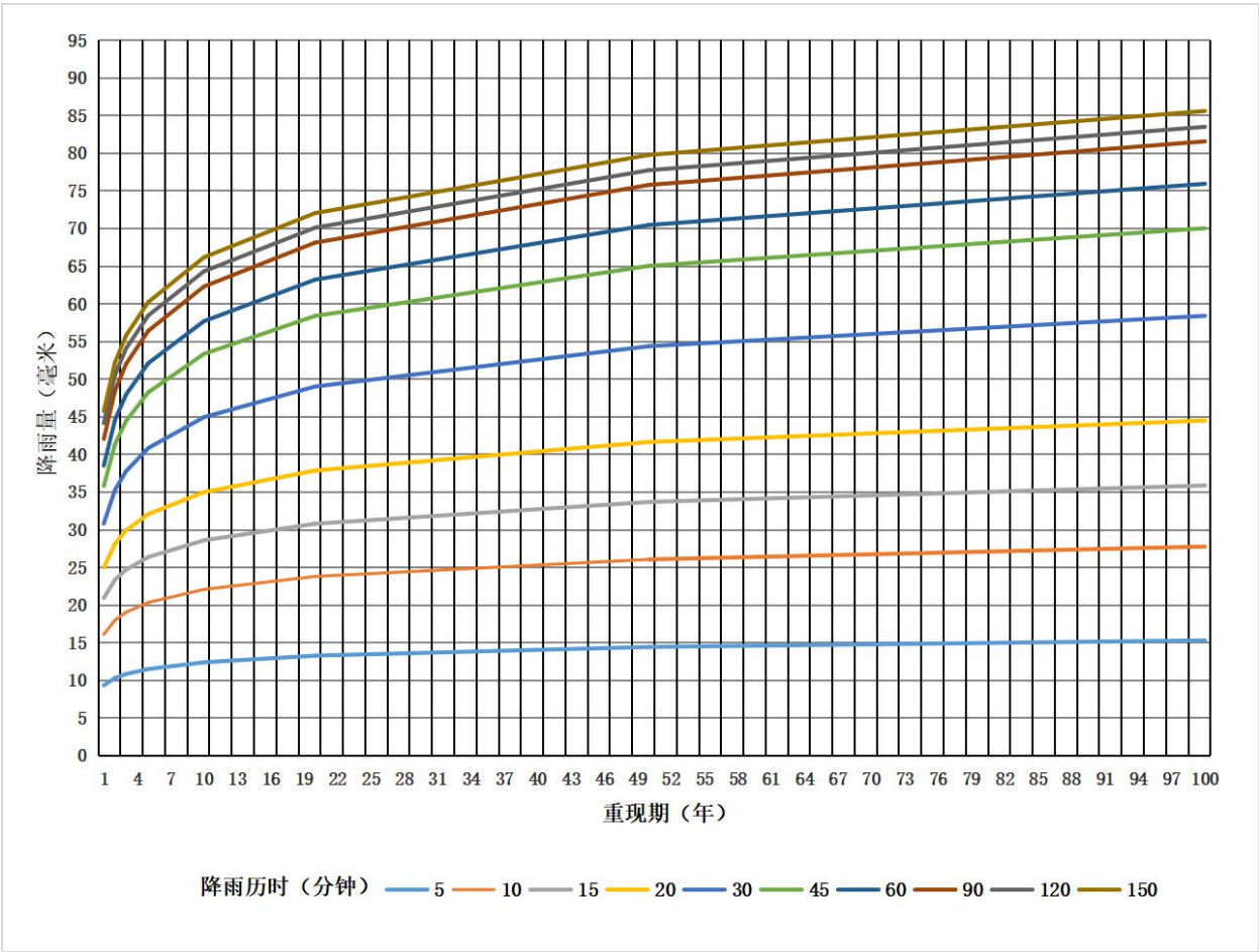
图 A.10 镇康县不同历时降雨曲线
