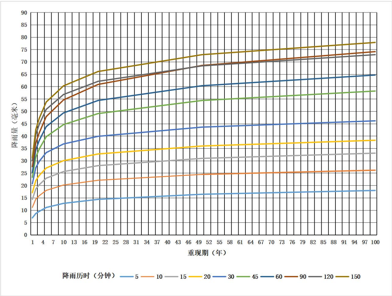
图 A.12 耿马县不同历时降雨曲线
