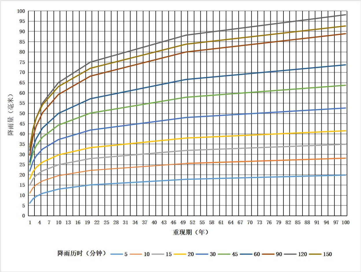
图 A.14 沧源县不同历时降雨曲线
