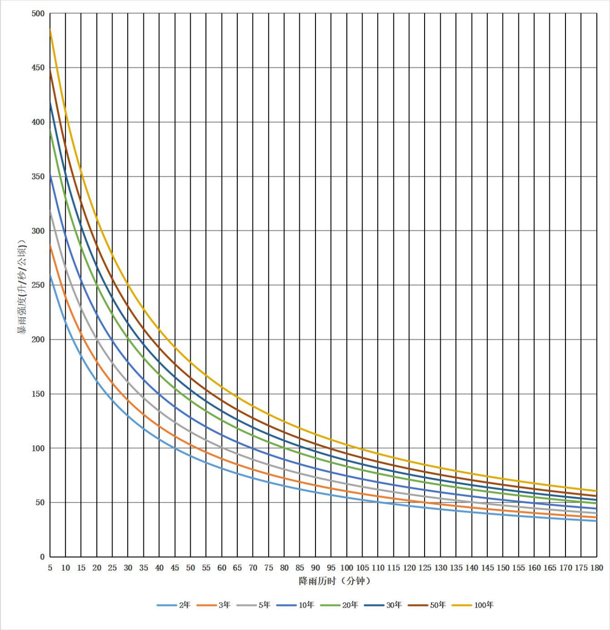
图 A.1 临翔区暴雨强度曲线
