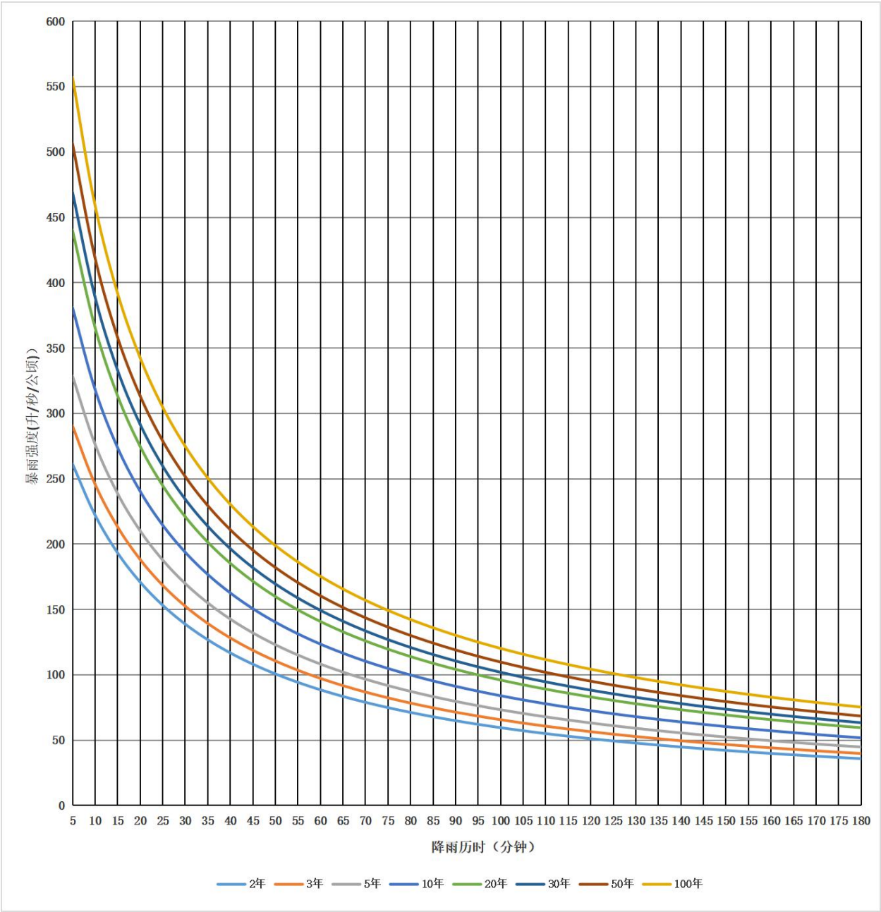
图 A. 7 永德县暴雨强度曲线
