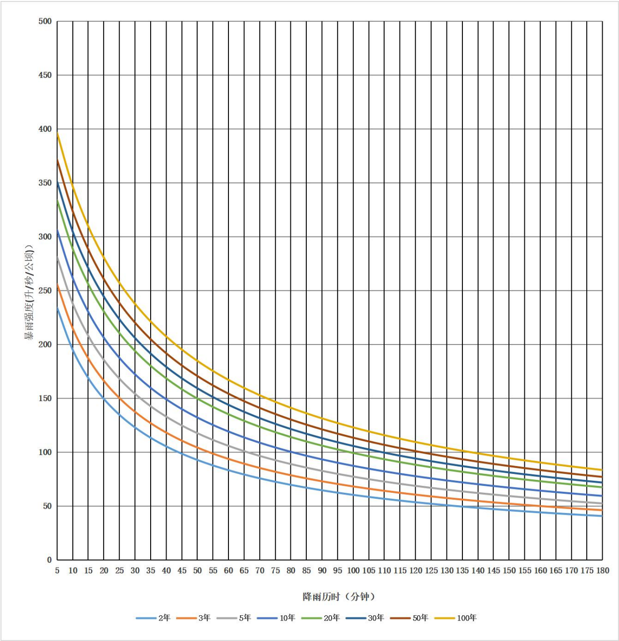
图 A.5 凤庆县暴雨强度曲线
