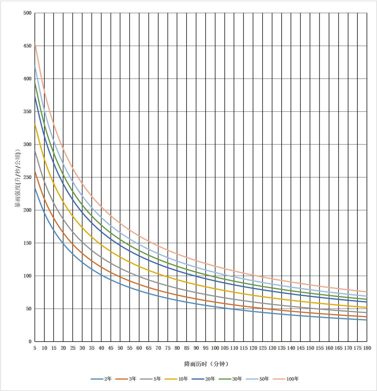
图 A.3 云县暴雨强度曲线
