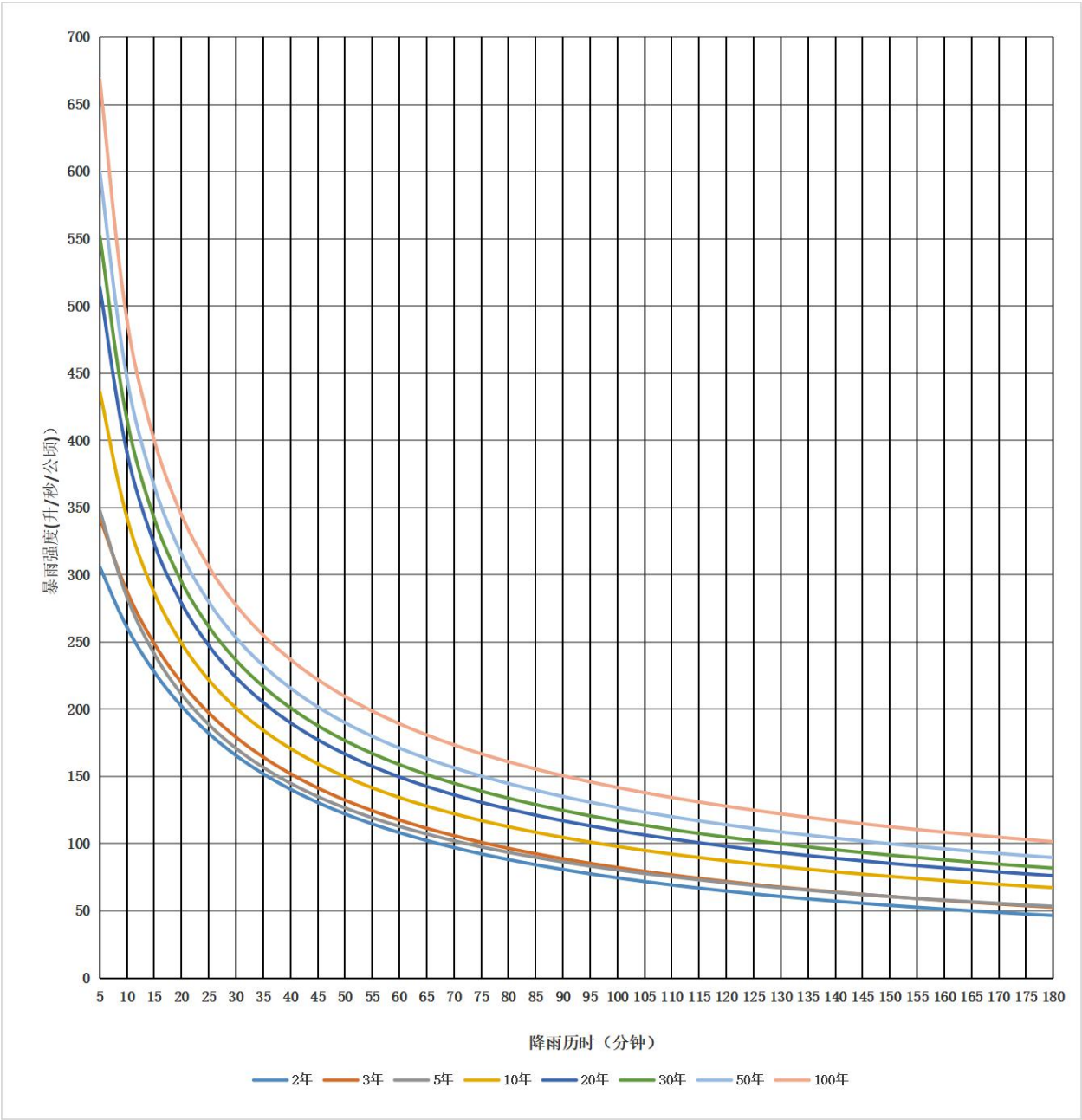
图 A. 13 沧源县暴雨强度曲线
