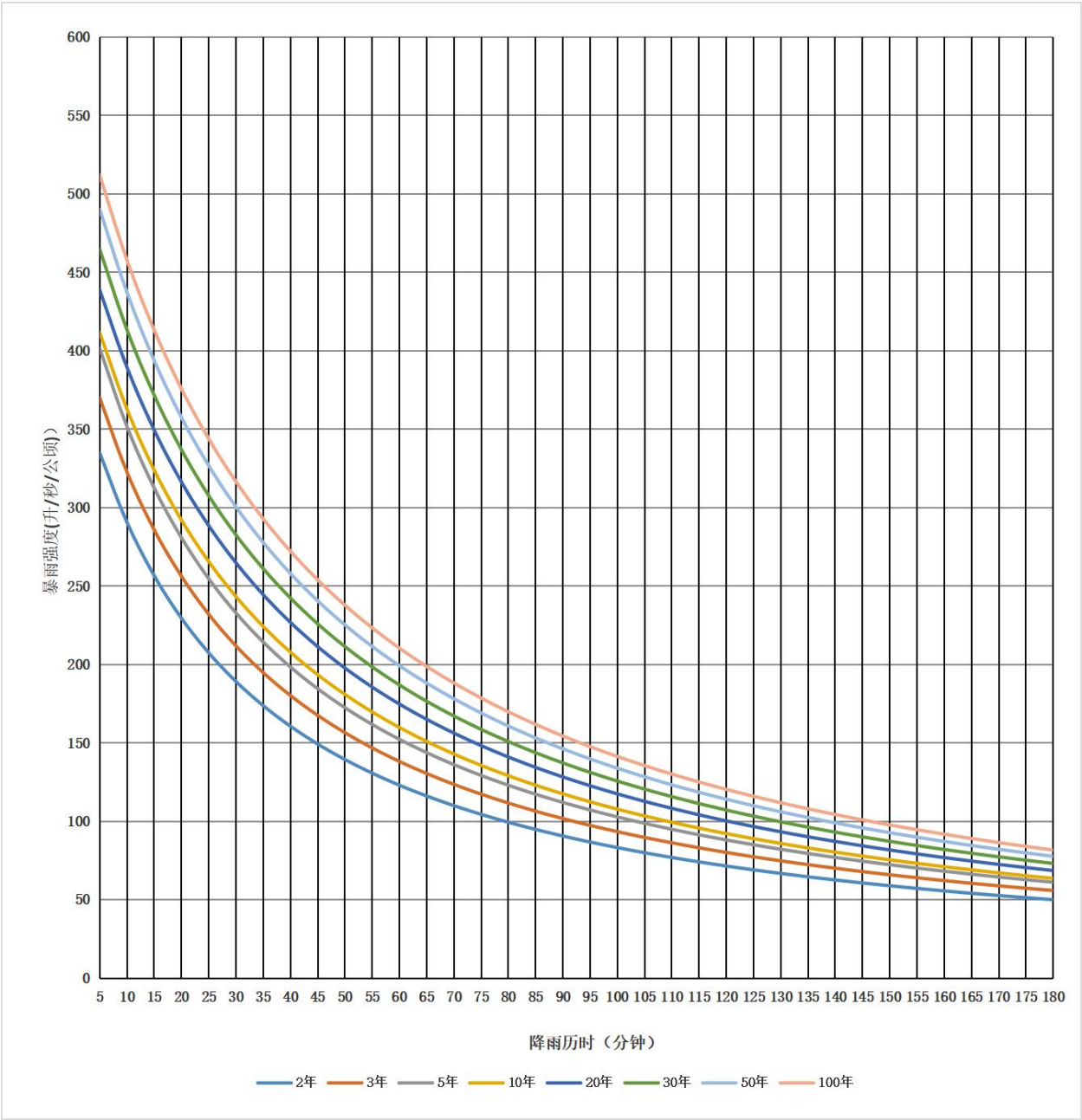
图 A. 9 镇康县暴雨强度曲线
