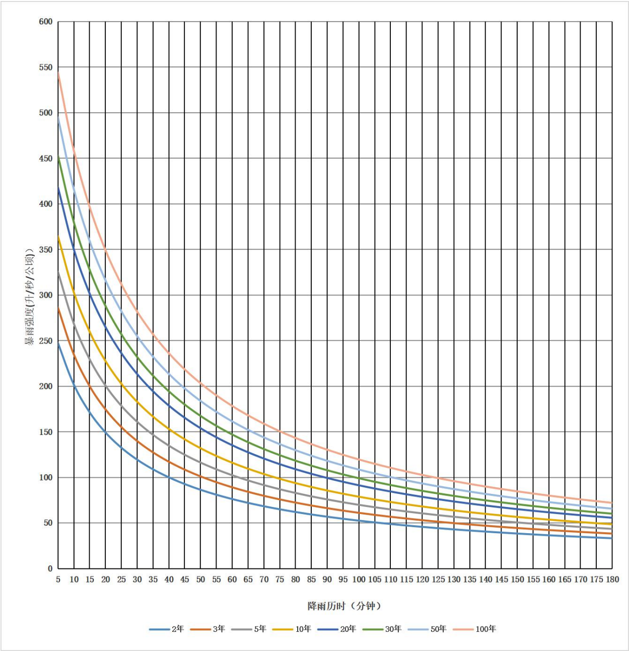
图 A. 15 双江县暴雨强度曲线
