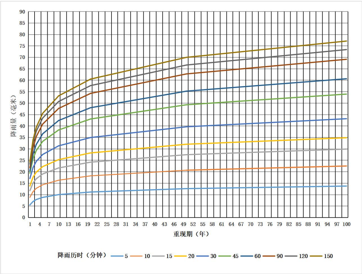
图 A. 4 云县不同历时降雨曲线
