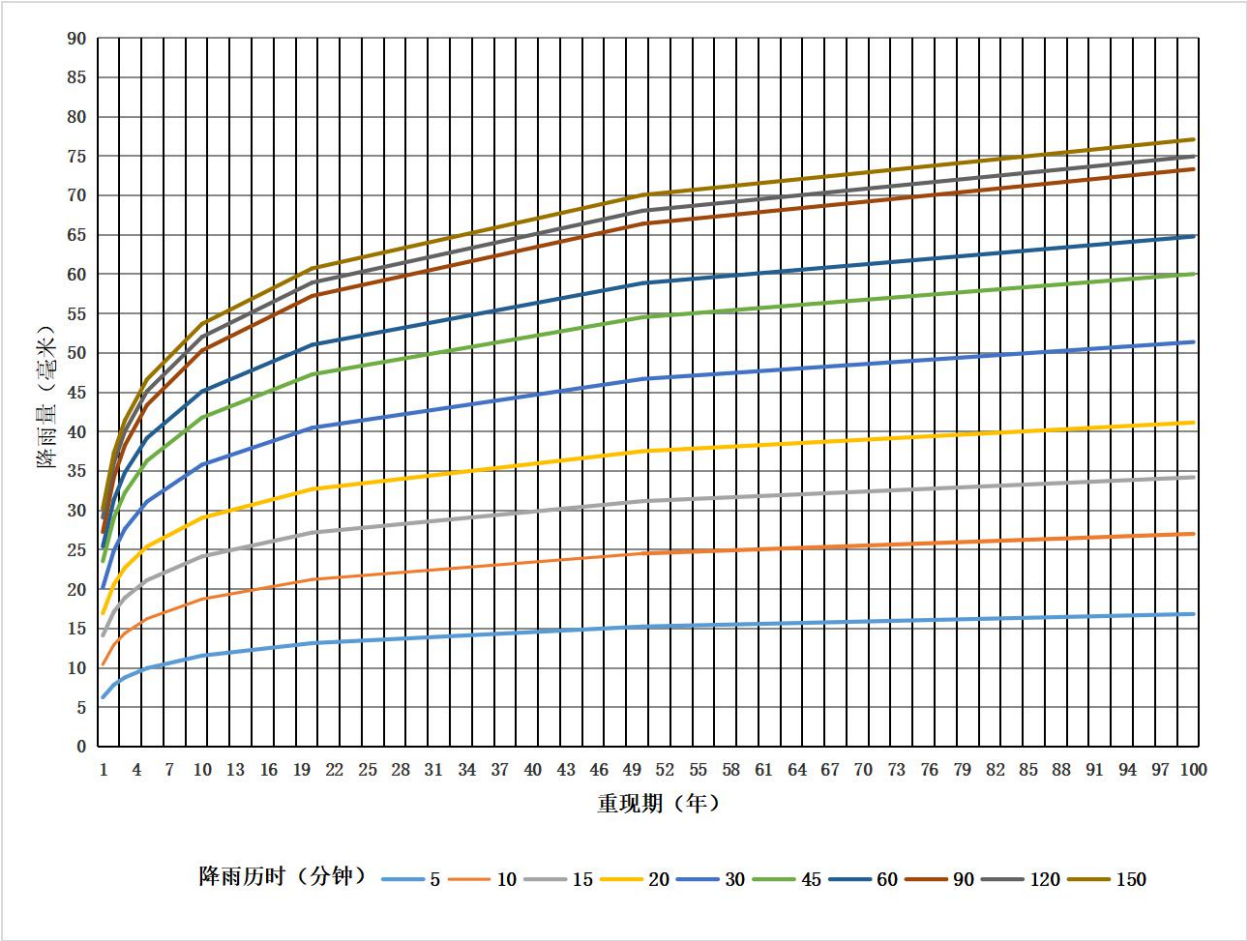
图 A. 8 永德县不同历时降雨曲线
