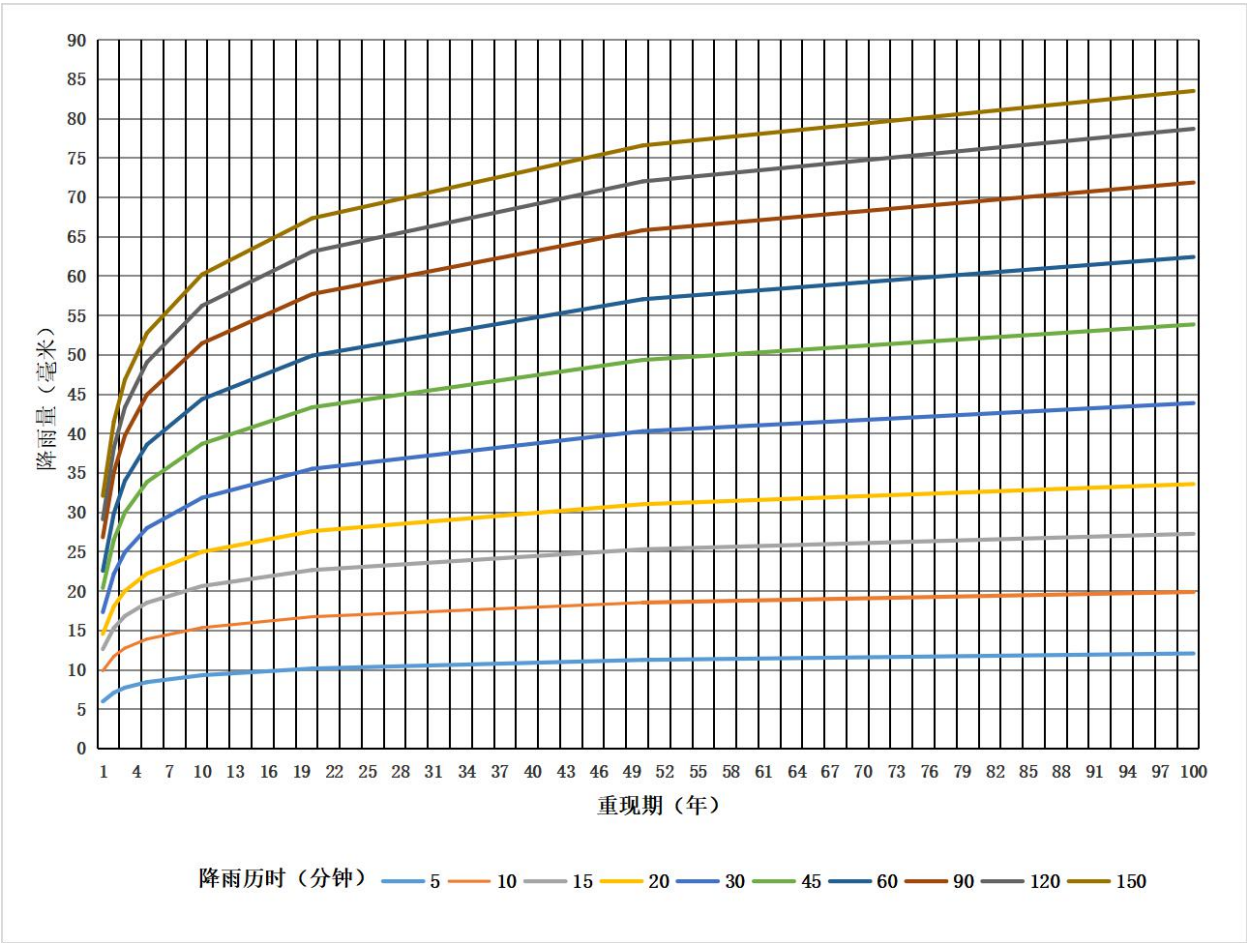
图 A. 6 凤庆县不同历时降雨曲线
