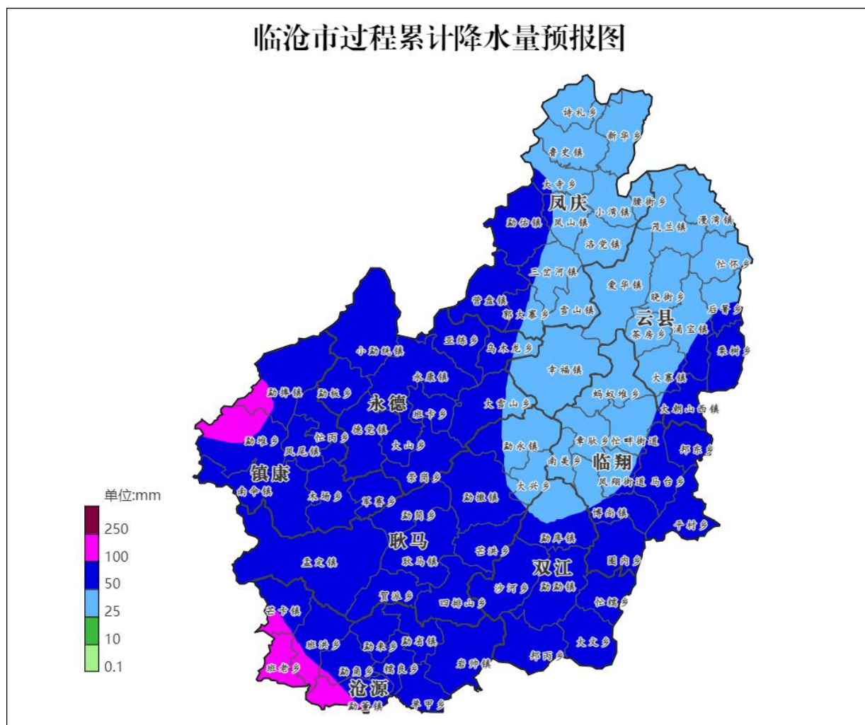
5月24日20时—28日20时降水量预报图（单位：毫米）
