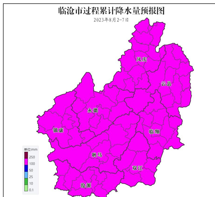
临沧市 2023 年 8 月 2—7 日降水量预报图（单位：毫米）
